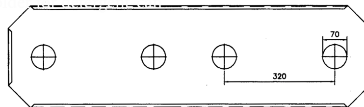
STANDARD DOUBLE FIXED BOTTOM 0,8 mm
